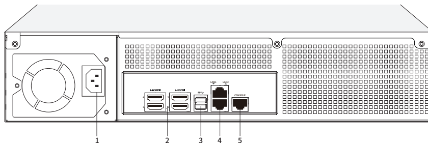
图1-4 TL-TUMS2700后面板示意图
