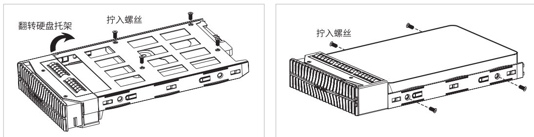
图3-3 2.5寸/3.5寸硬盘安装硬盘
