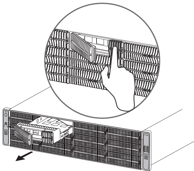
图3-2 抽出硬盘盒
